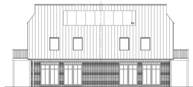
Ansicht West Villa Wattkicker
