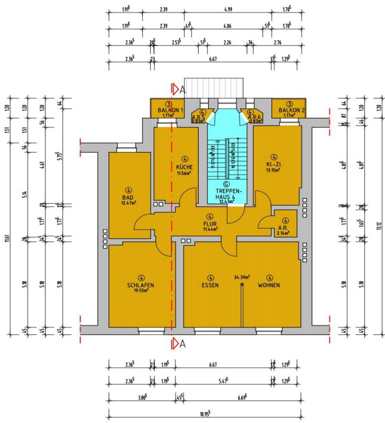
2. OBERGESCHOSS
