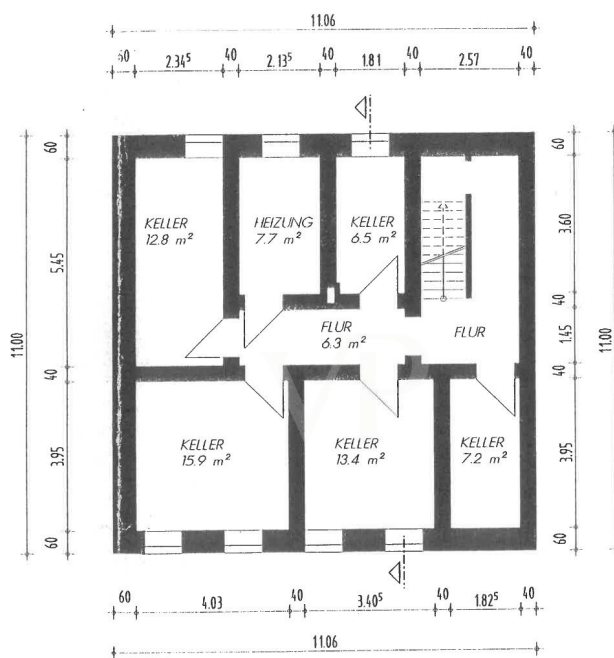
KELLERGESCHOSS
