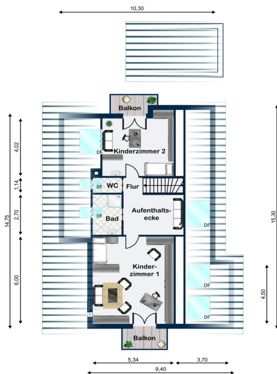
Dachgeschoss
