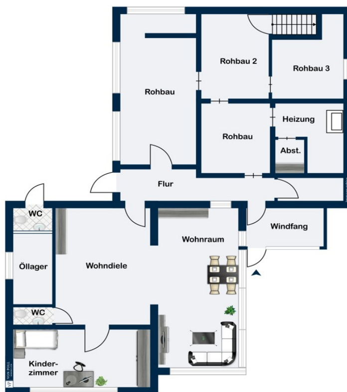
Untergeschoss
