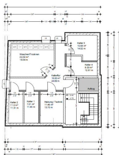
Kellergeschos
