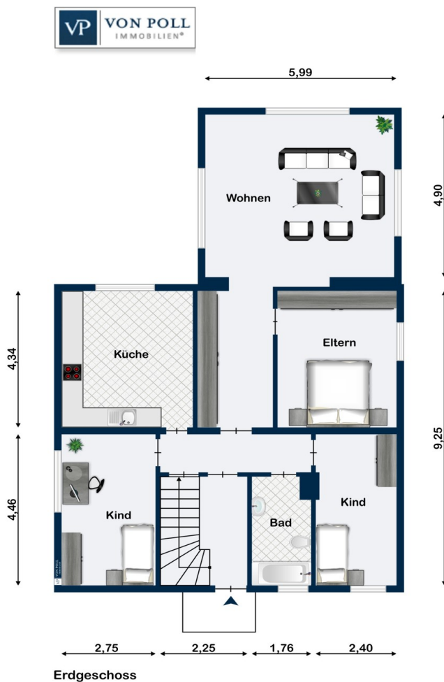
Erdgeschoss
