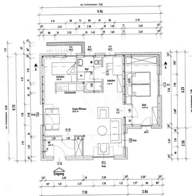
Erdgeschoss M 1:50
