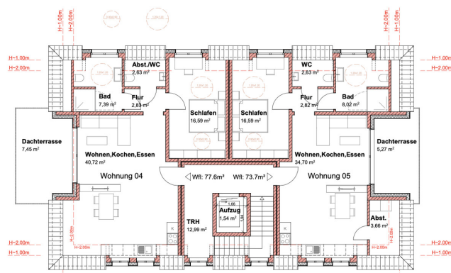
GRUNDRISS DG
