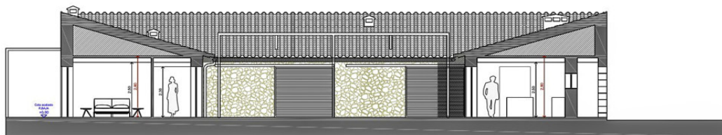
SECCIÓN 2 E: 1/150
