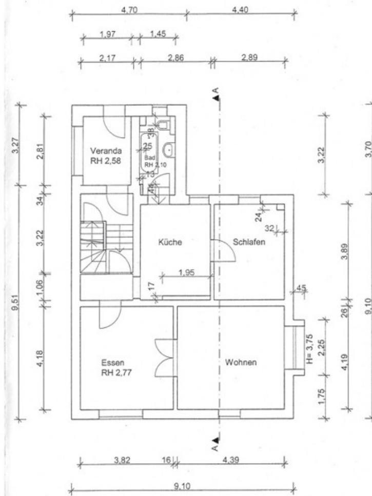
Grundriss Erdgeschoss
