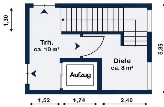
Obergeschoss
