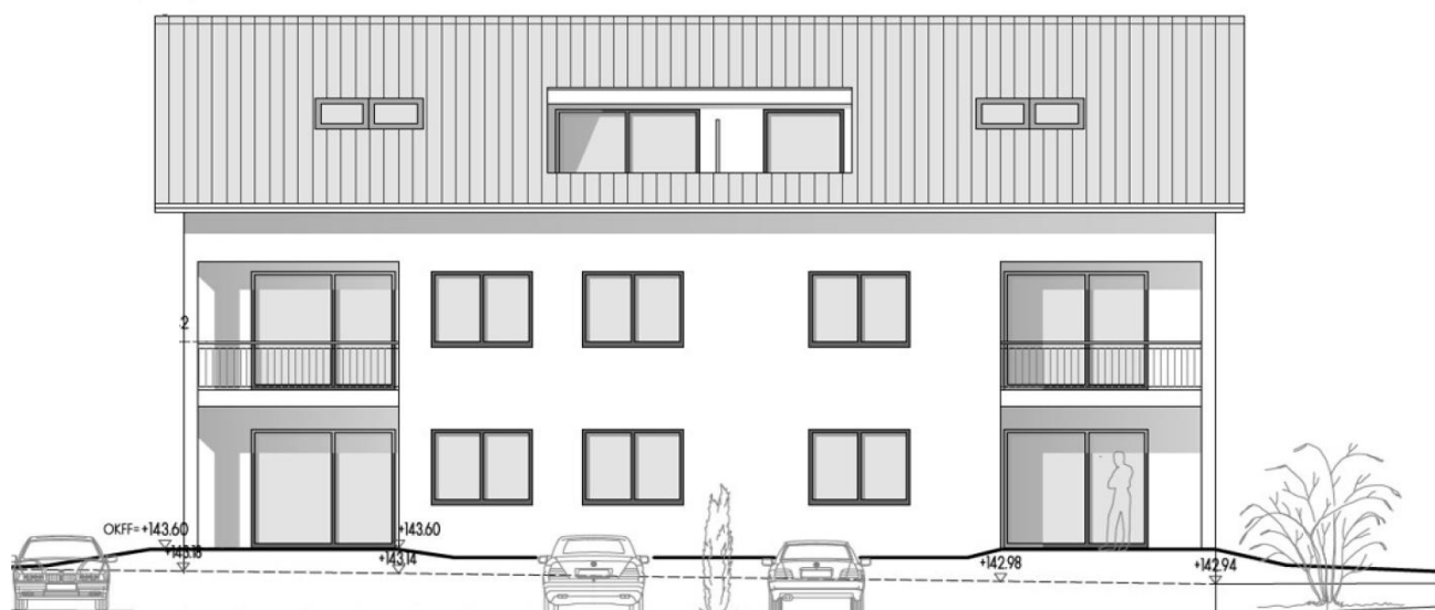
Süd - West - Ansicht
