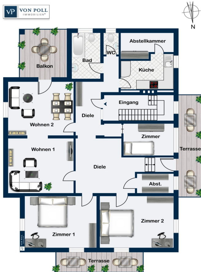
1. Obergeschoss
