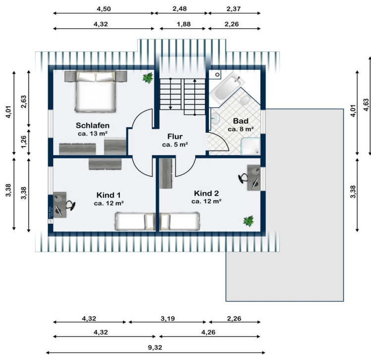
Dachgeschoss
