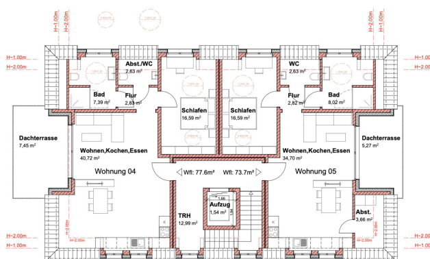
GRUNDRISS DG
