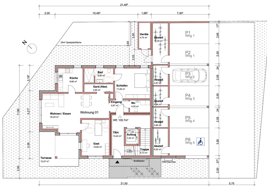
GRUNDRISS EG
