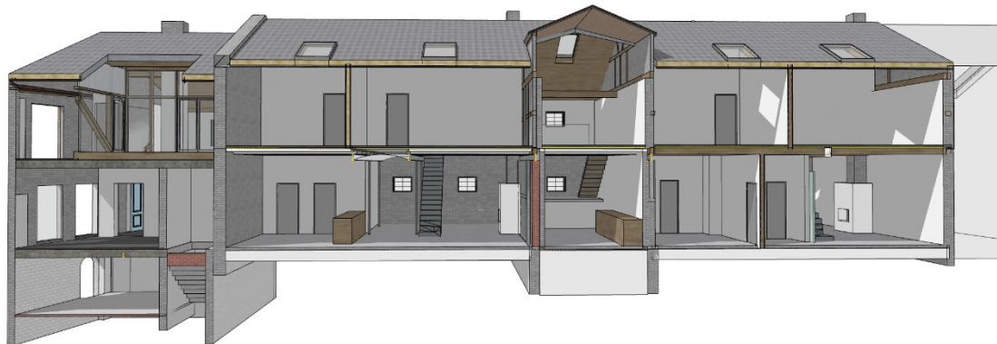
Längsschnitt Anbau & Stallspeicher, Blick von Süden
