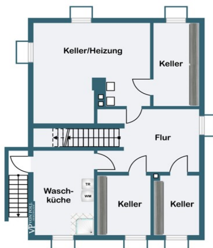
Kellergeschoss
