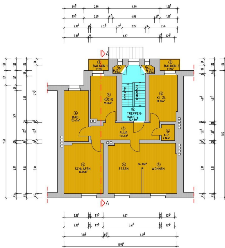
2.OBERGESCHOSS
