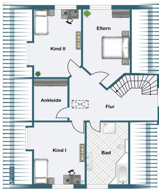
Dachgeschoss
