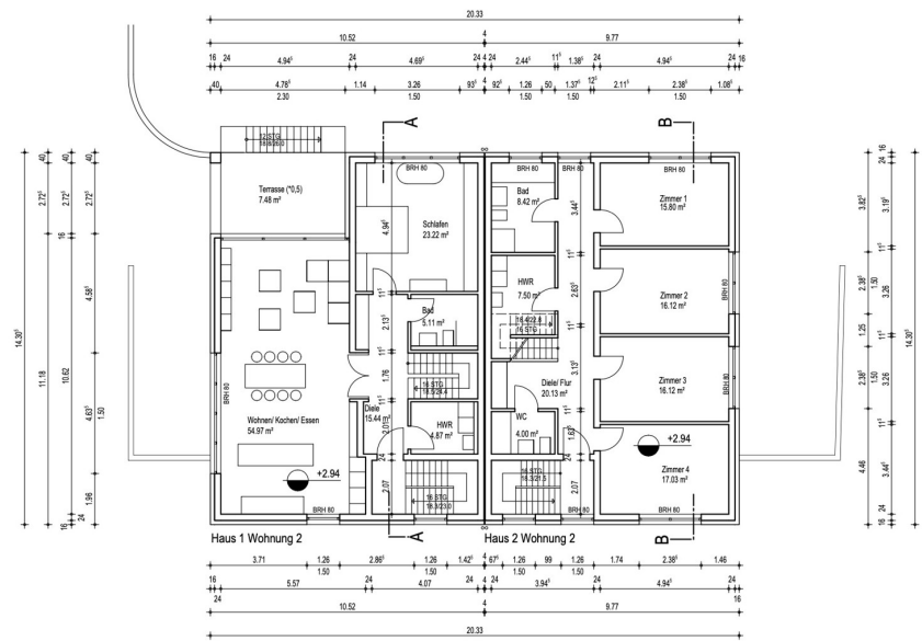
Obergeschoss
