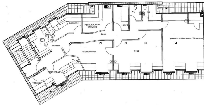
GRUNDRISS 2. OBERGESCHOSS
