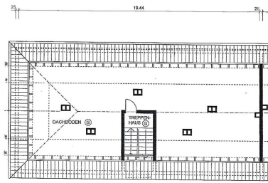
Grundris Dachboden
