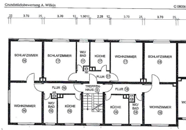
Grundris 1. Obergeschoss (unmaßstäblich) des Mehrfamilienhauses Lohengrinstraße 7
