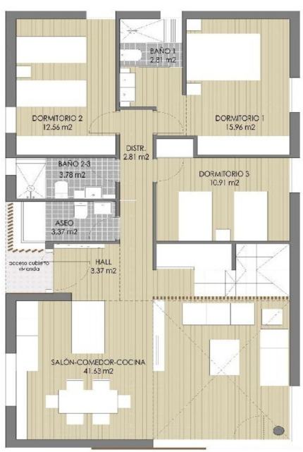
PLANTA BAJA
