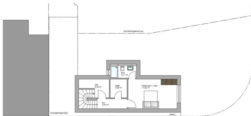
KELLERGESCHOSS EFH WOHFÄCHE ca. 11,06m² NUTZFÄCHE ca. 4,13m²
