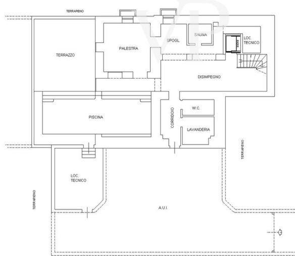
PIANO SOTTOSTRADA 1 (H=2,70)
