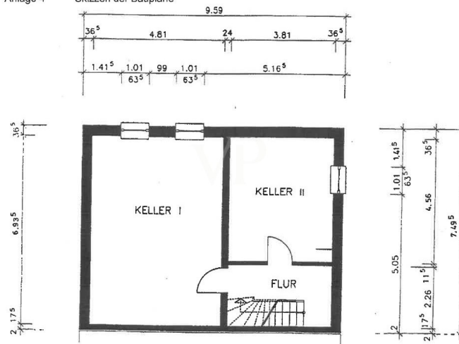
Anlage 4 Skizzen der Baupläne
