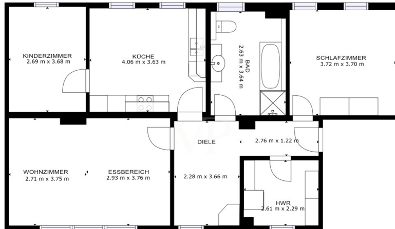
1. OBERGESCHOSS
