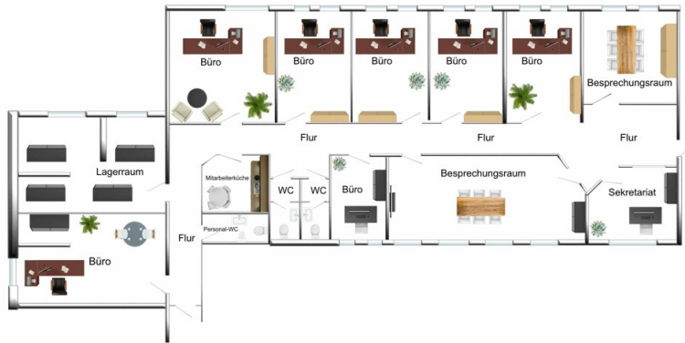
Dachgeschoss
