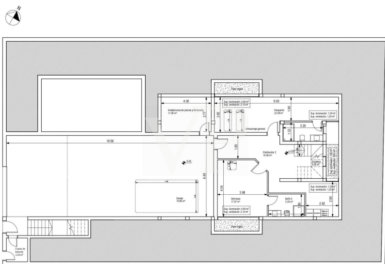
PLANTA SÓTANO
