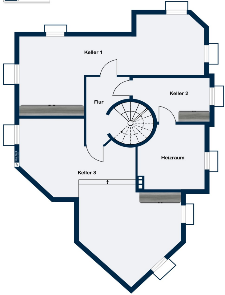
Kellergeschoss
