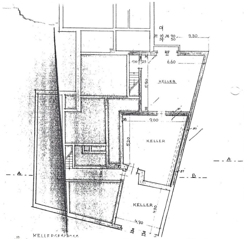
KELLERGESCHOSS
