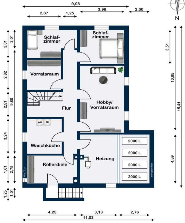
Kellergeschoss
