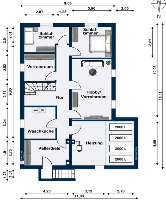
Kellergeschoss
