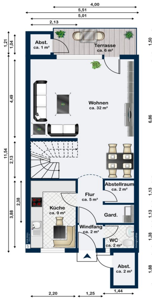
Erdgeschoss
