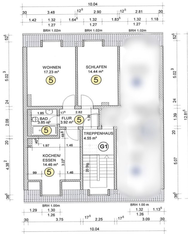
DACHGESCHOSS 5 = 53.90 m²
