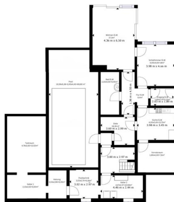
Gartenebene Gesamtfläche ca. 223,74 m 2
