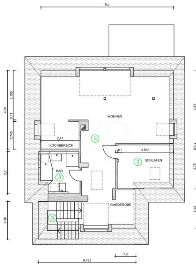
GRUNDRISS DACHGESCHOSS
