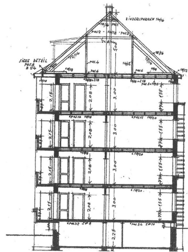
Schnittzeichnung
