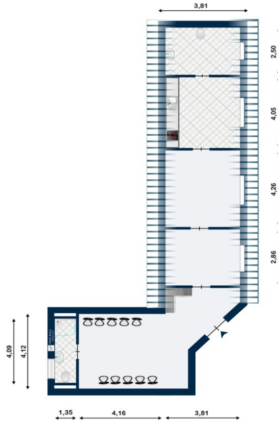
Mezzanin
