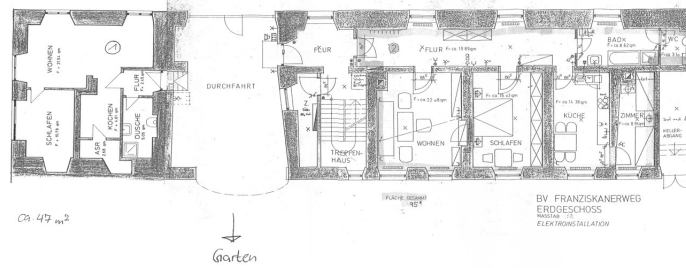
Erdgeschoss
