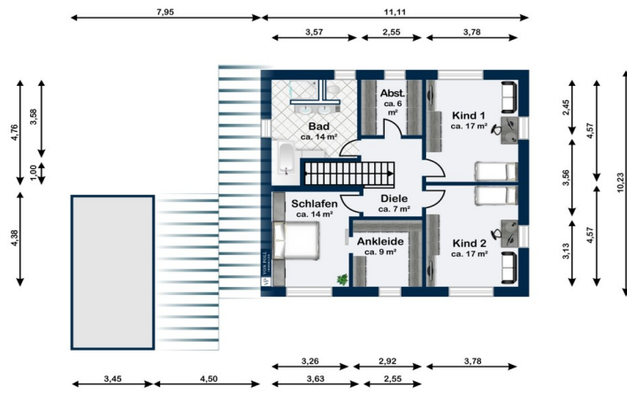
Obergeschoss
