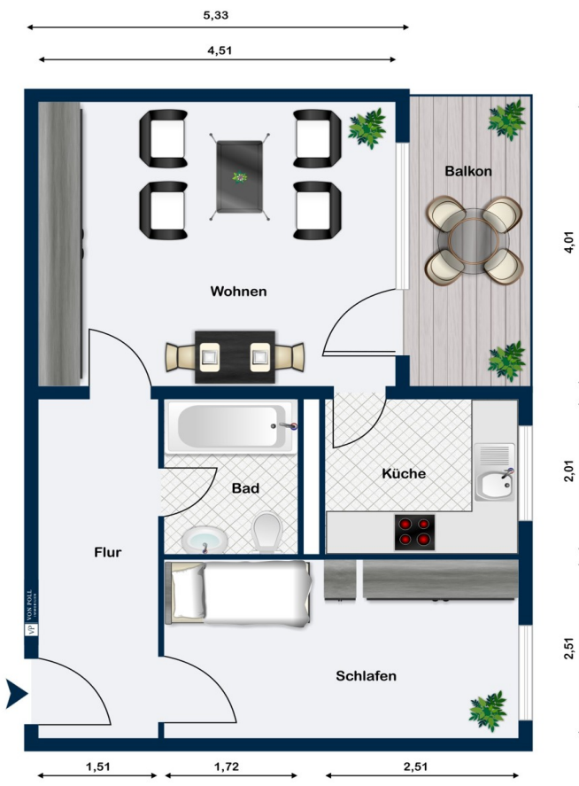
4. Obergeschoss
