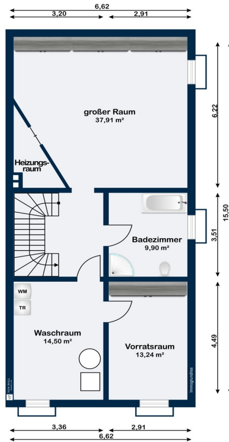
Kellergeschoss
