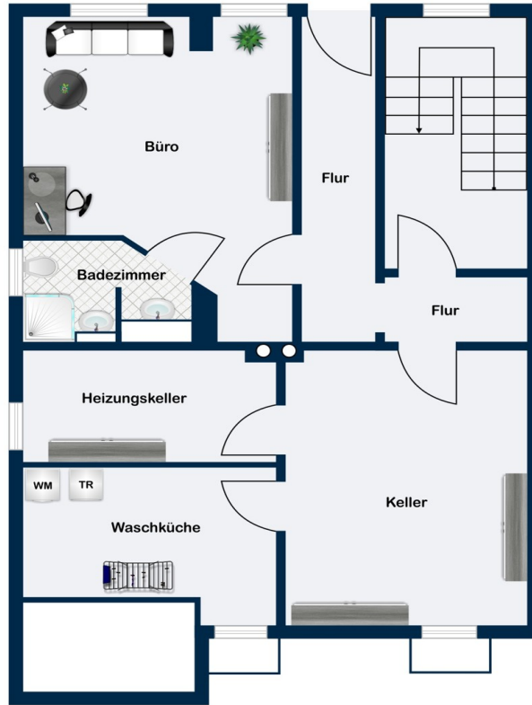
Kellergeschoss
