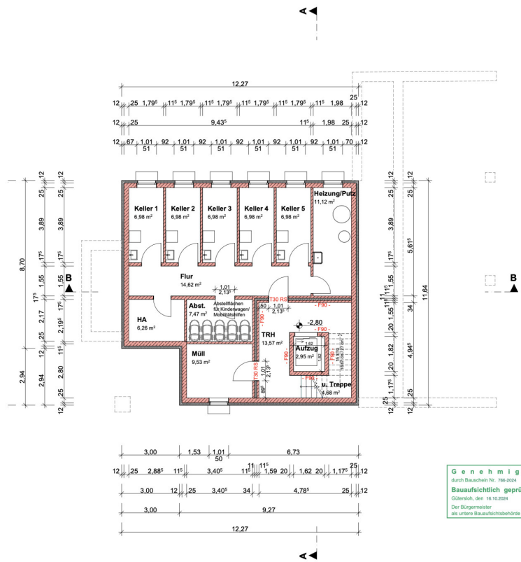
GRUNDRISS UG
