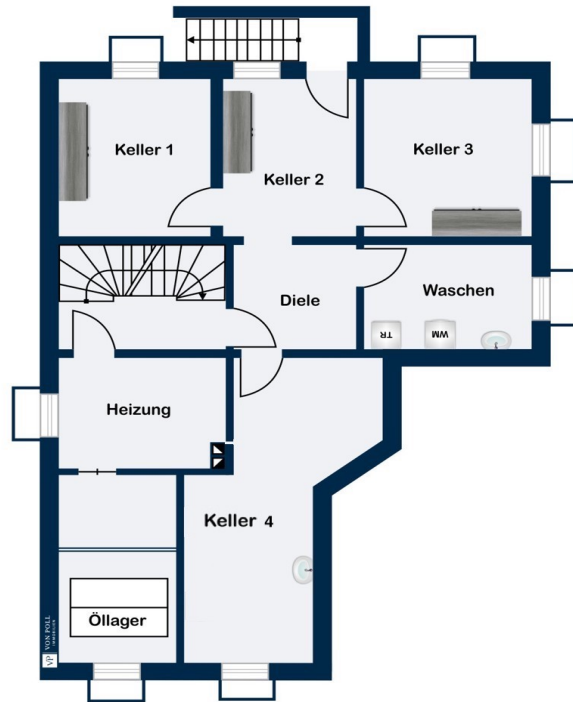
Kellergeschoss
