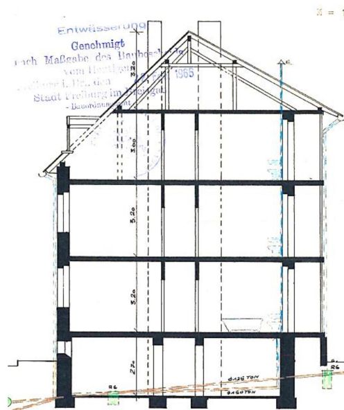
Gebäudeschnitt Vorderhaus
