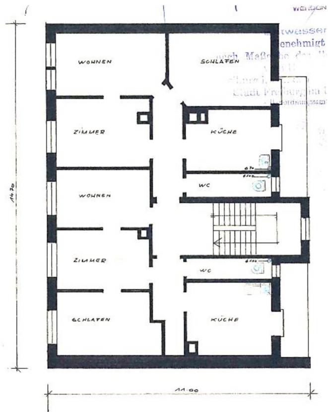
Obergeschoss Vorderhaus
