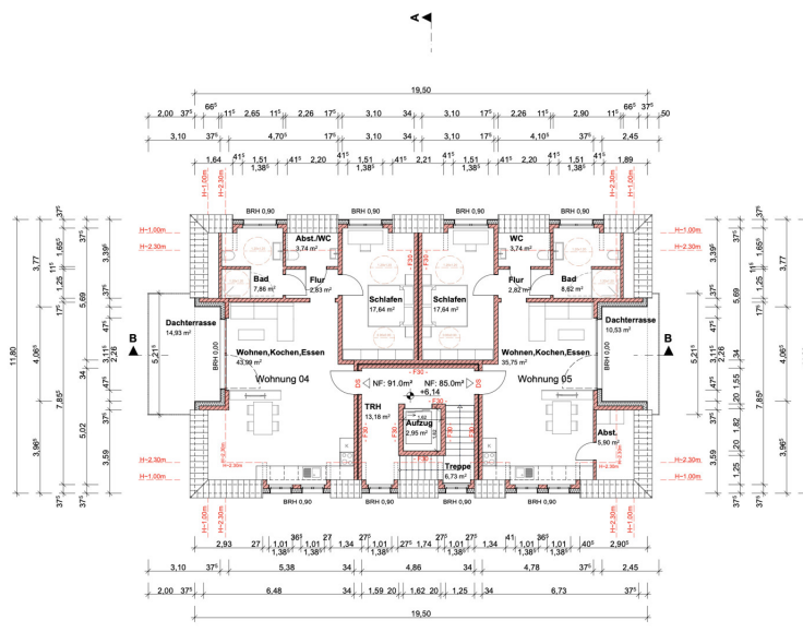
GRUNDRISS DG
